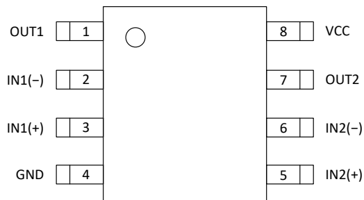
TSSOP-8
