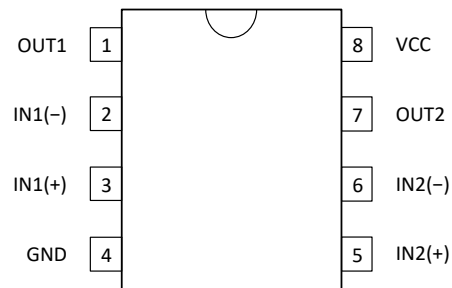
DIP-8
