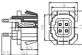
パネル取付穴寸法参考図 適合シャーシ厚 t1.6
